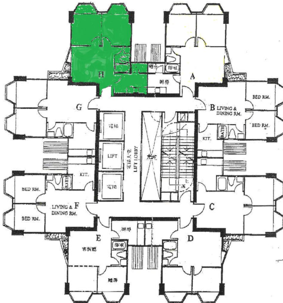
5樓至34樓平面圖
